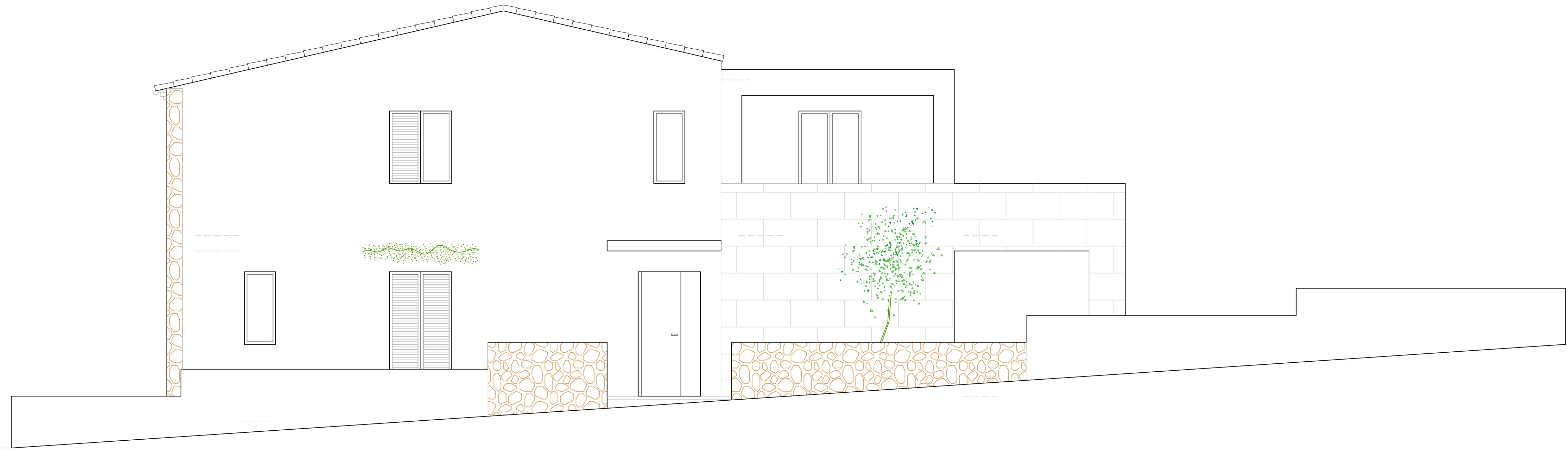
ALZADO POSTERIOR
