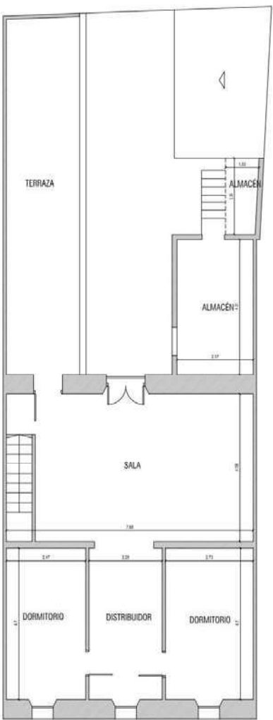
PLANTA PISO SUP. CONSTRUIDA: 99,30M2
