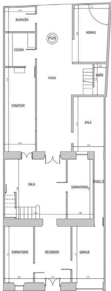
PLANTA BAJA SUP. CONSTRUIDA: 140,80M2
