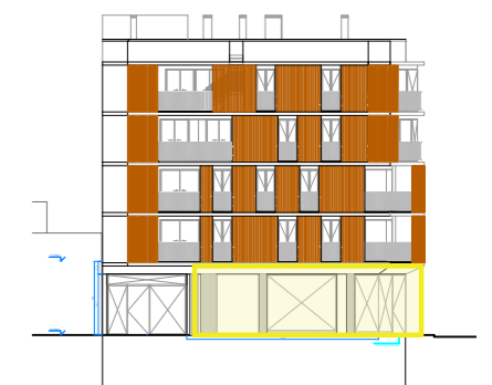
Alzado calle Foners
