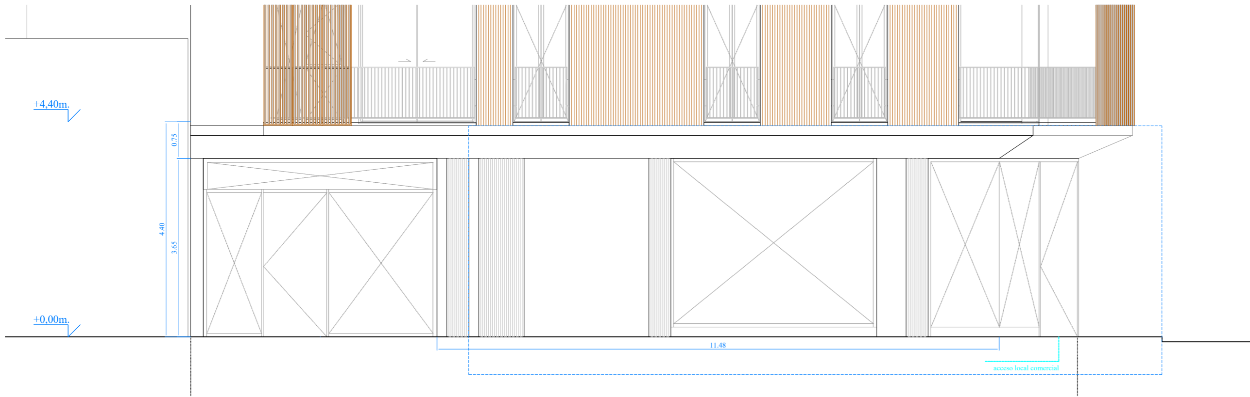
Alzado calle Foners
