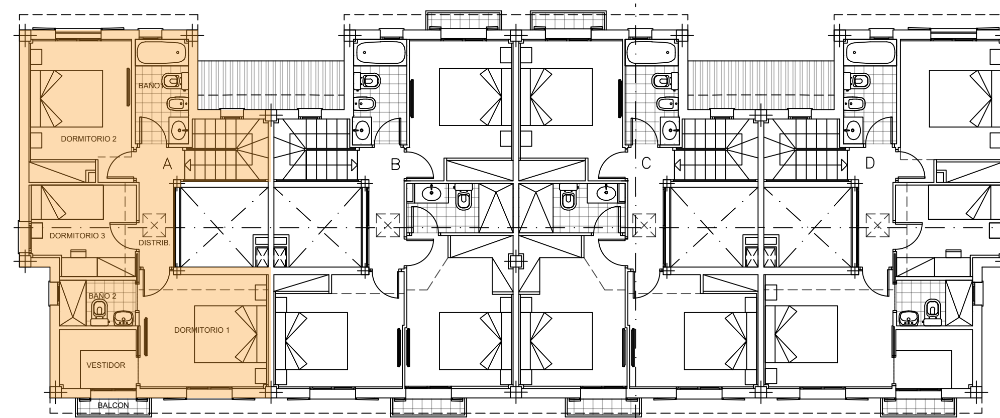
PLANTA ALTA
