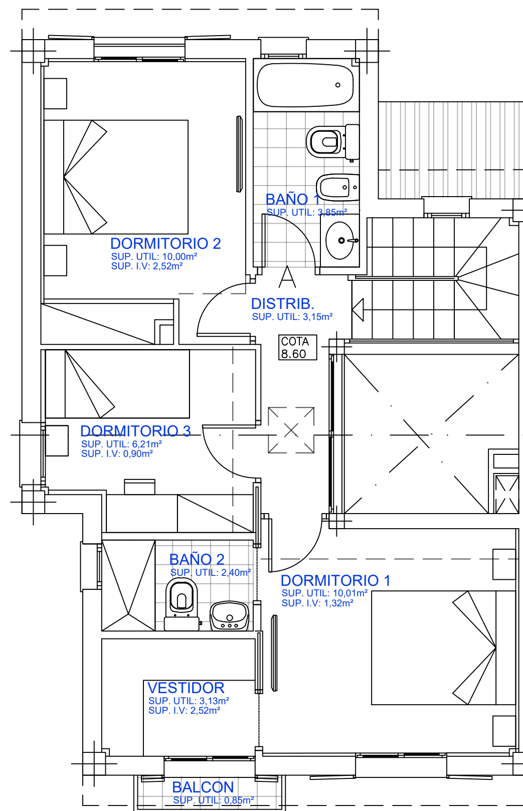
PLANTA ALTA
