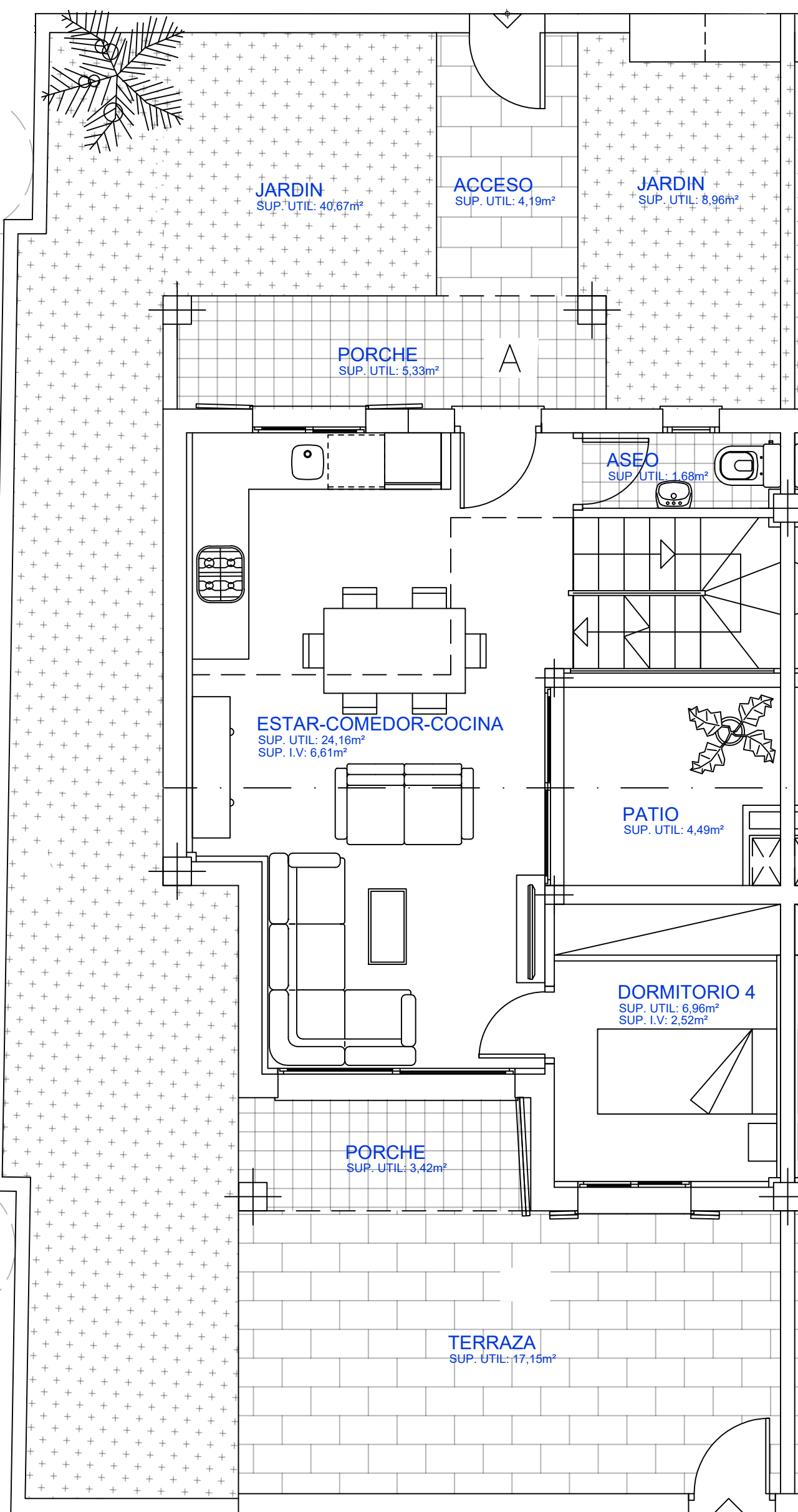
PLANTA BAJA
