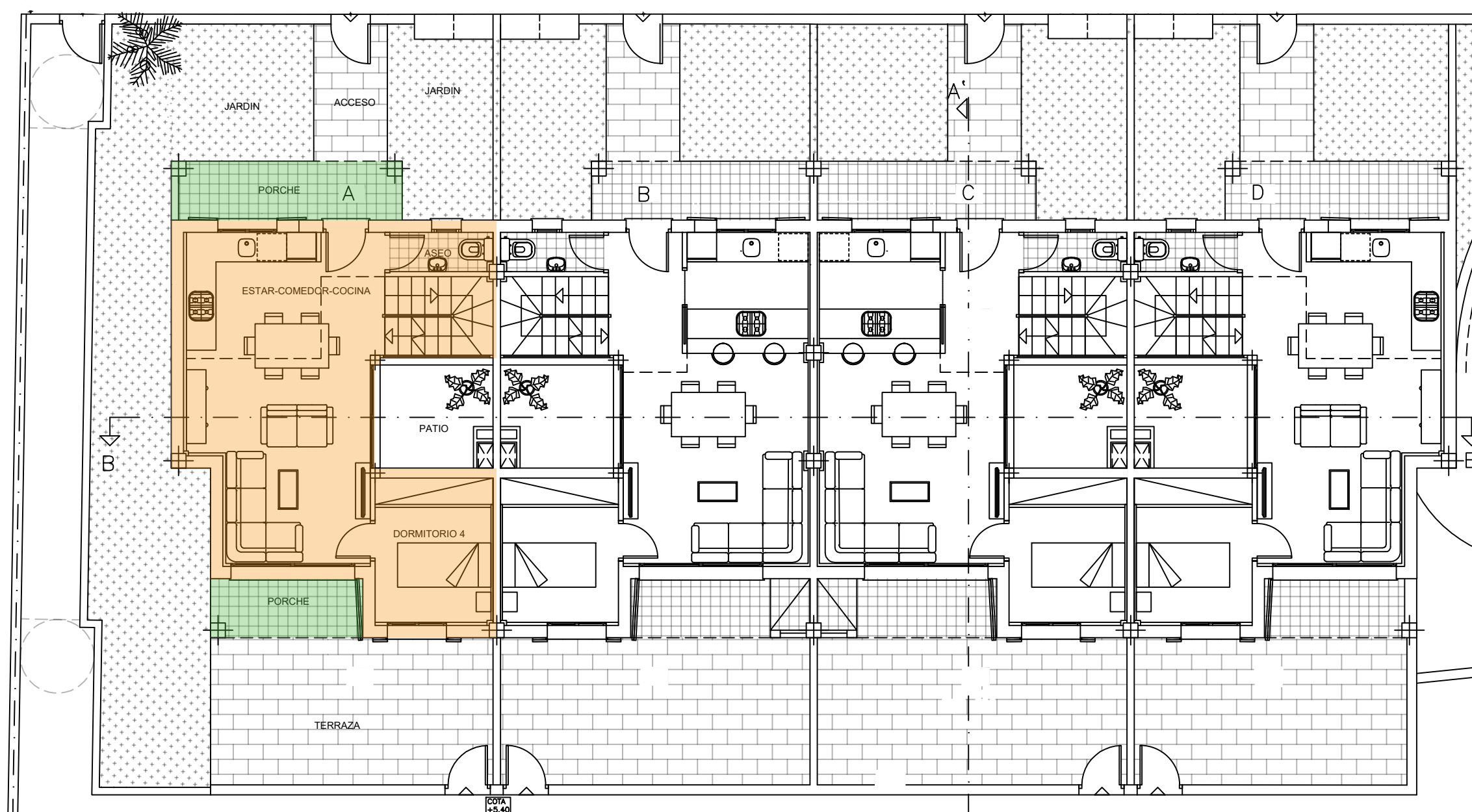
PLANTA BAJA
