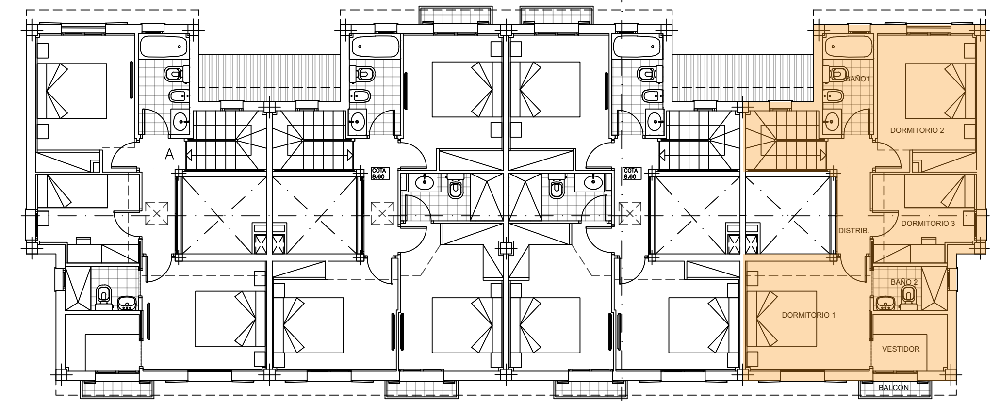
PLANTA ALTA
