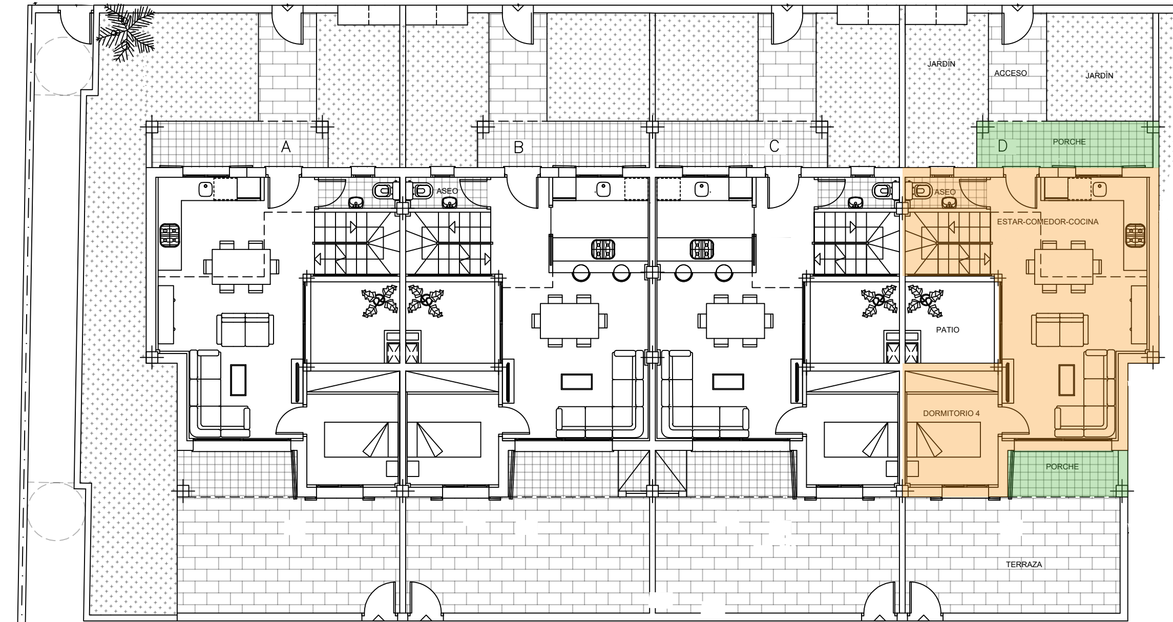
PLANTA BAJA
