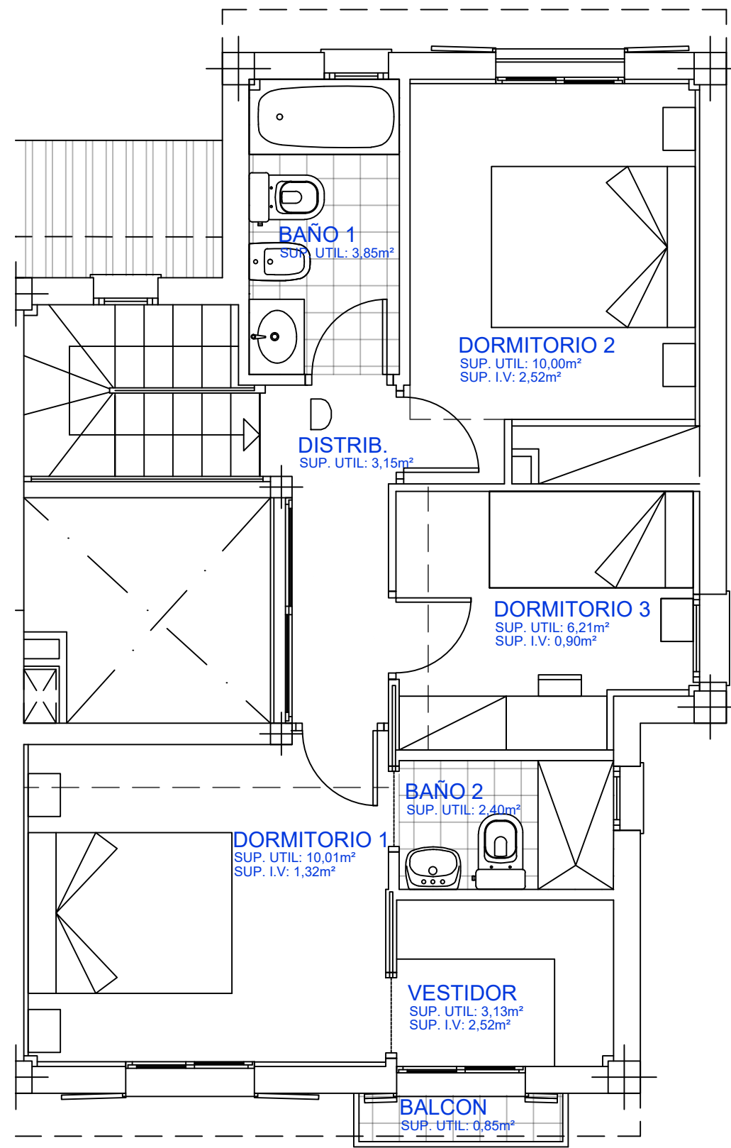
PLANTA ALTA
