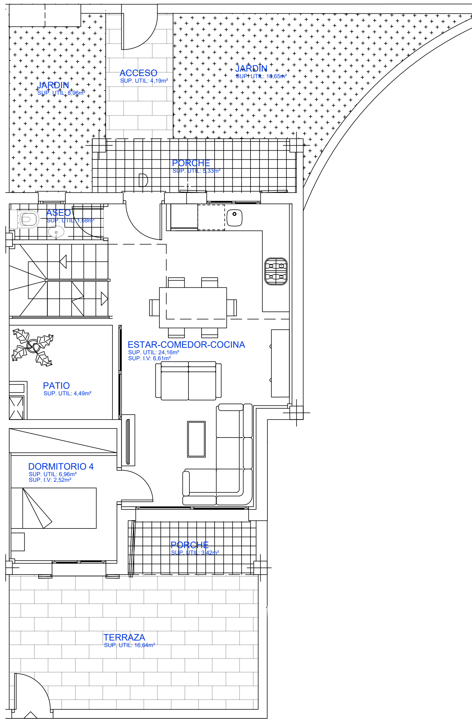
PLANTA BAJA
