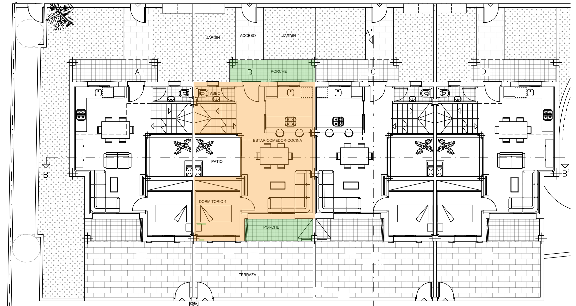
PLANTA BAJA
