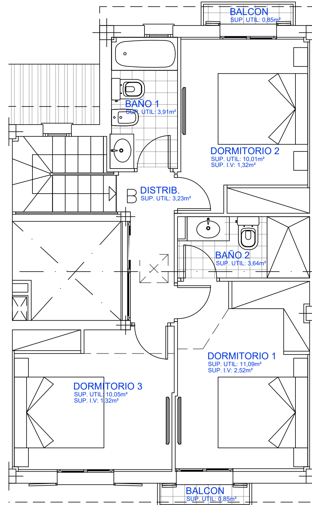
PLANTA ALTA
